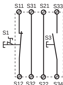
Fig. 3: Circuito de entrada monocal, rearme supervisado/Circuito di ingresso monocal, start controllato/Eenkanalig ingangscircuit, bewaakte start
