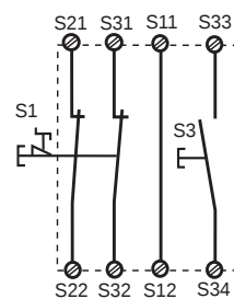
Fig. 4: Circuito de entrada bicanal, rearme supervisado/Circuito di ingresso bicanal, start controllato/Tweekanalig ingangscircuit, bewaakte start
